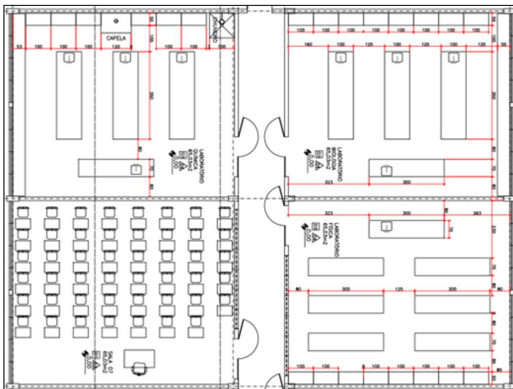
Figura 02. Layout dos laboratórios de biologia, química, física e de uma sala de aula.
