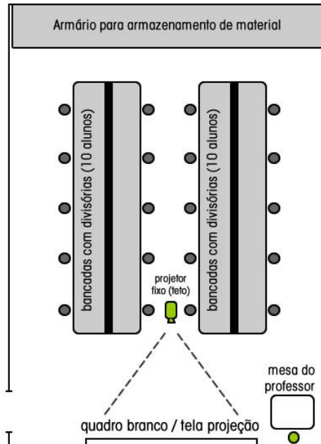
Figura 6 - Layout de laboratório de Instalação e Manutenção de Computadores / Redes com capacidade para 20 estudantes
